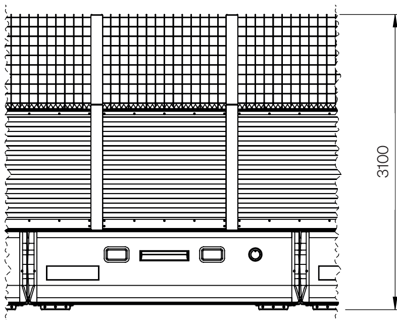
Toppnätsutförande
